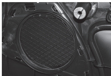
9. Emplacement dans la garniture de portière. Veillez à ce que la membrane ne vienne pas en contact avec la garniture.
